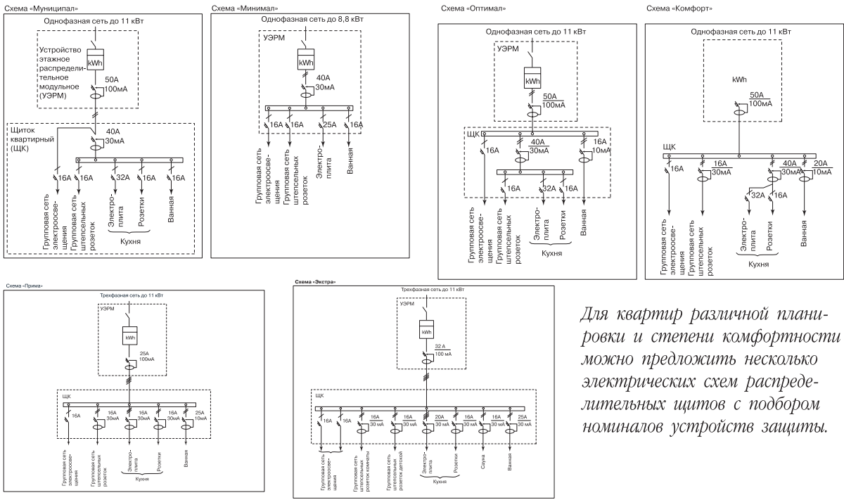
Схема подключения УЗО и автоматов
