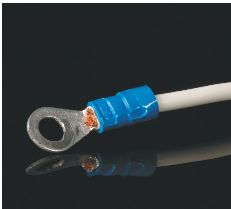
Наконечники на проводе закрепляются методом опрессовки или пайки.
